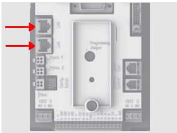
Рисунок 10: З'єднання Link
